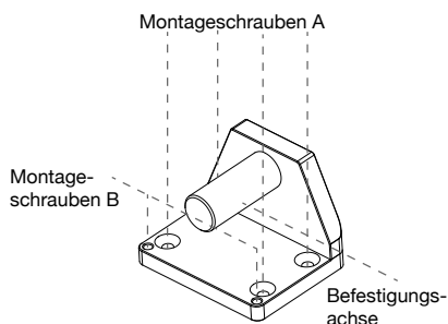
Montageplatte
